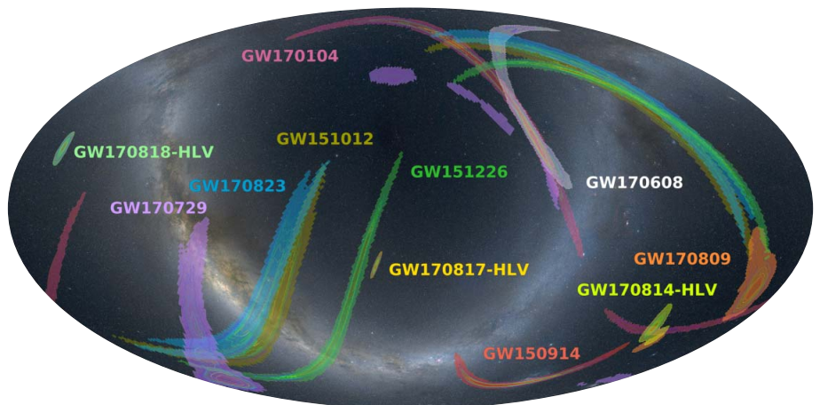
3. ábra. A LIGO O1–O2 megfigyelési időszakai alatt észlelt gravitációshullám-jelek forrásaihoz meghatározott éterületek, amelyeken belül történtek a kompakt objektumok összeolvadásai (forrás: LIGO-Virgo, Háttér: Axel Mellinger).
